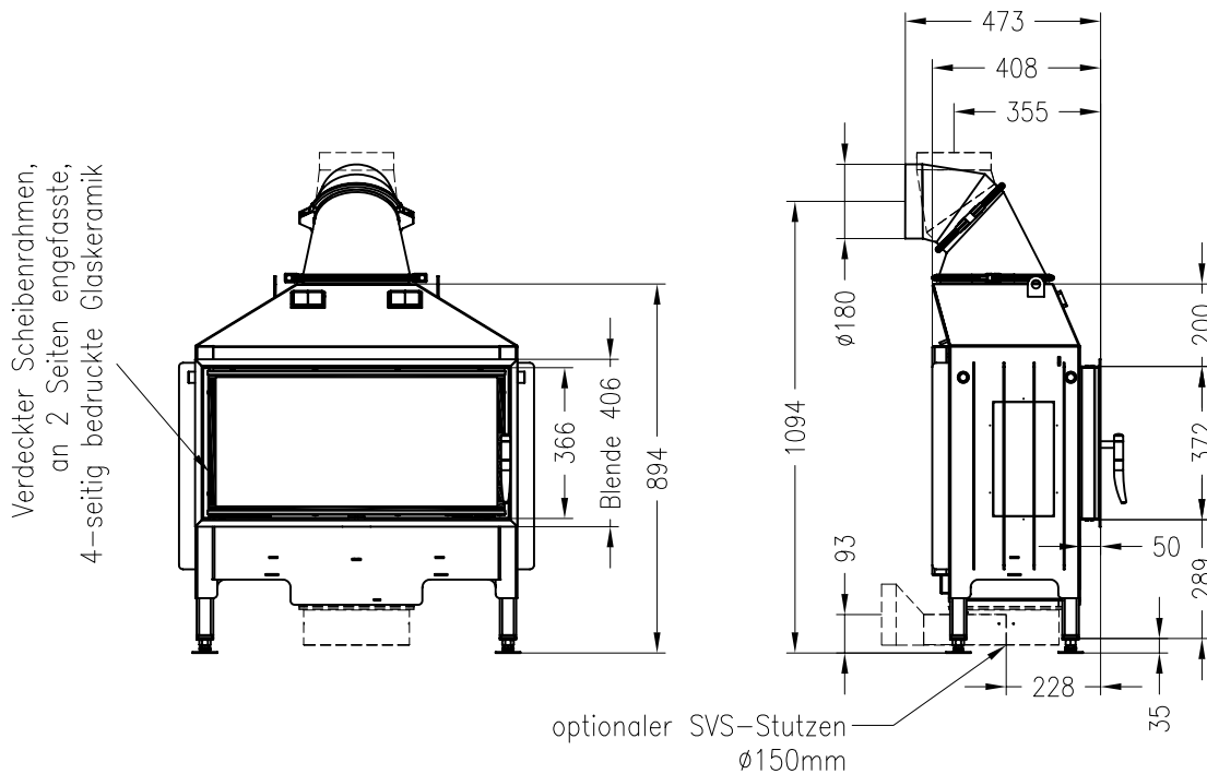
Vorderansicht M ~1:20
